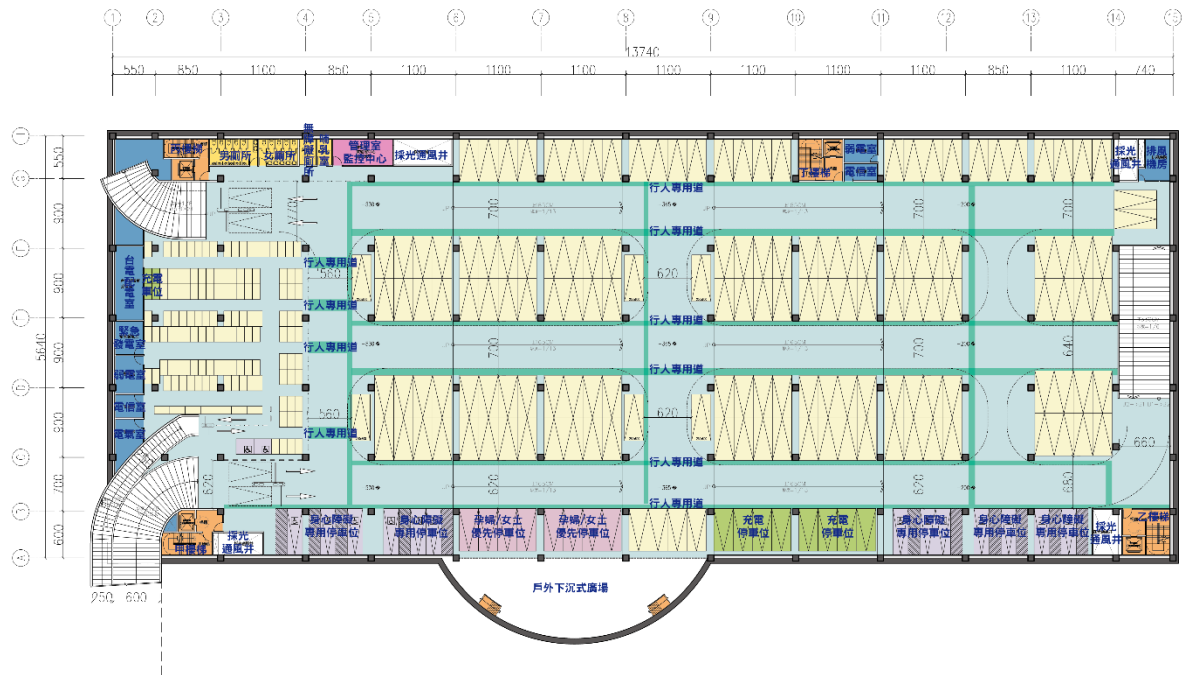
地下 2 樓平面示意圖(概念設計圖，僅供參考)
